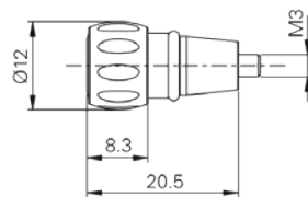
2622-1014 Feineinstellvorrichtung
