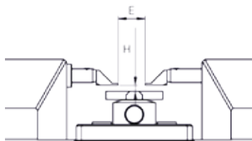
PS 15 - Auflagetisch XYZ 1362-1005 E: Messweg 10 mm
